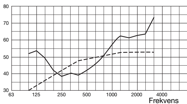
Dn,e (dB) ljudreduktion
